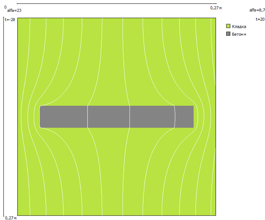
Рисунок 3 – Температурное поле неоднородного участка конструкции. Линии равной температуры проходят с шагом 4 °C начиная с -24 °C и заканчивая 16 °C.
